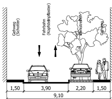
Schnitt M-M': Küsterstraße
