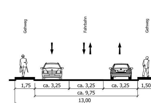
Schnitt G-G': Rolandstraße - B431
