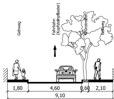
Schnitt L-L': Riststraße
