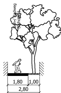
Schnitt B-B': Jungfernstieg
